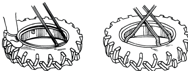
Рис. 2-35. Демонтаж шины
