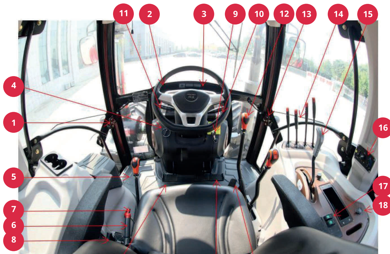
Рис. 2-1. Ручные органы управления и педали
