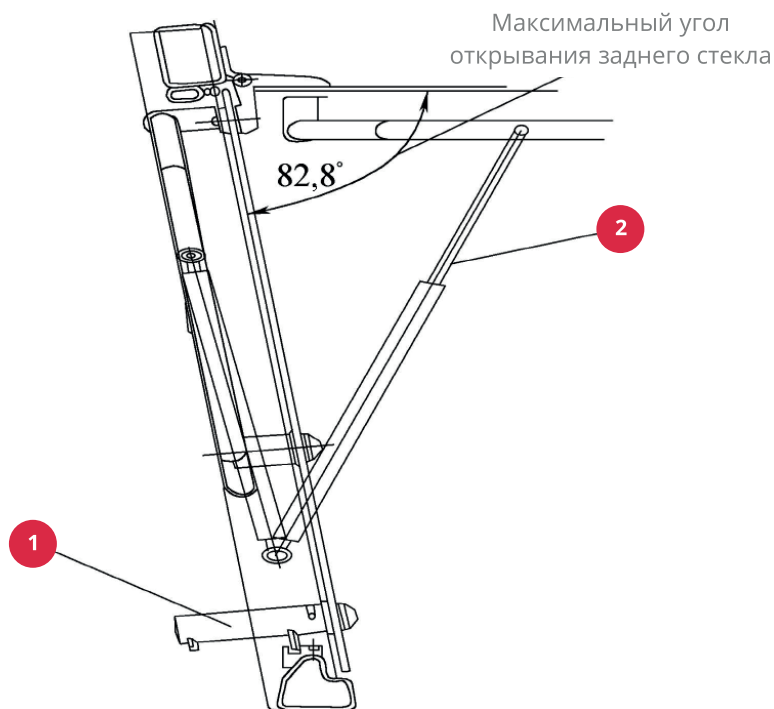
Рис. 2-49. Заднее стекло
