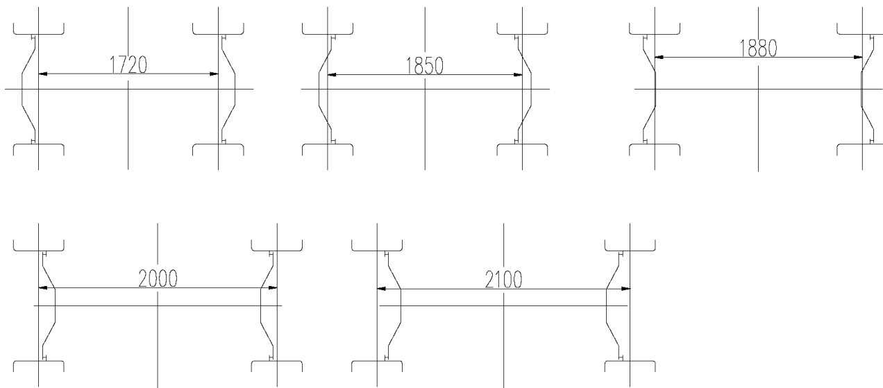
Рис. 2-30. Варианты ширины колеи передних колес
