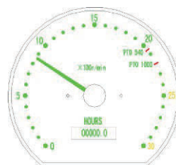
Рис. 2-4. Тахометр
