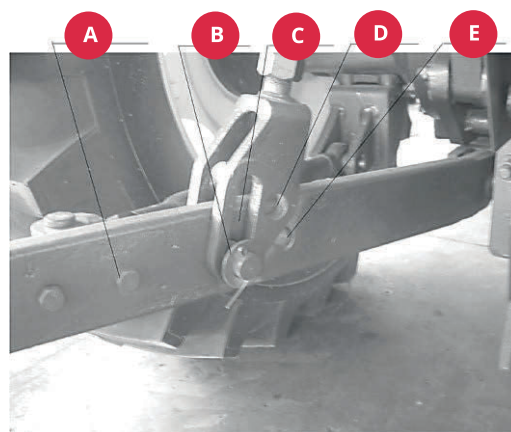
Рис. 2-71. Нижняя тяга
