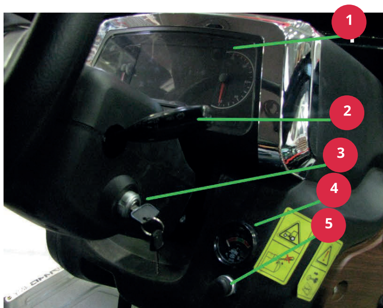
Рис. 2-2. Комбинация приборов и подрулевые переключатели
