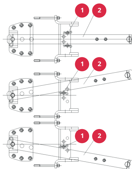
Рис. 3-1. Отклонение тягового бруса
