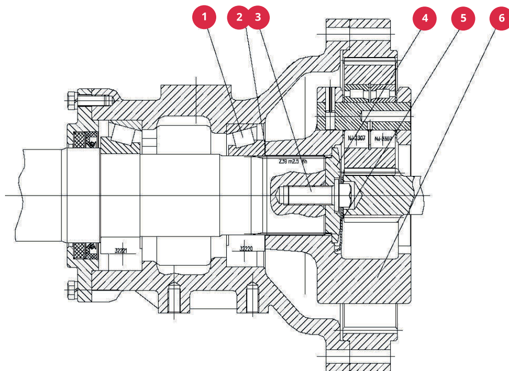
Рис. 4-24. Колесный редуктор
