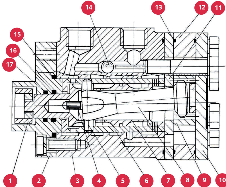
Рис. 4-28. Рулевой механизм
