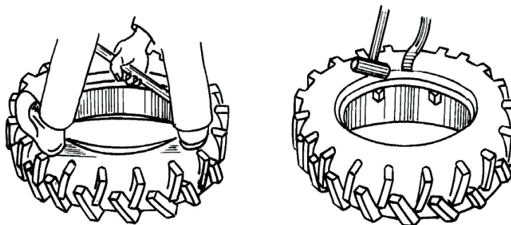
Рис. 2-36. Монтаж шины
