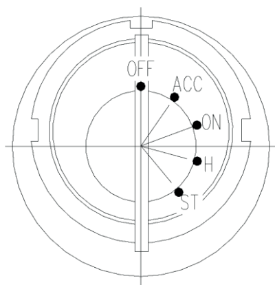
Рис. 2-18. Замок зажигания
