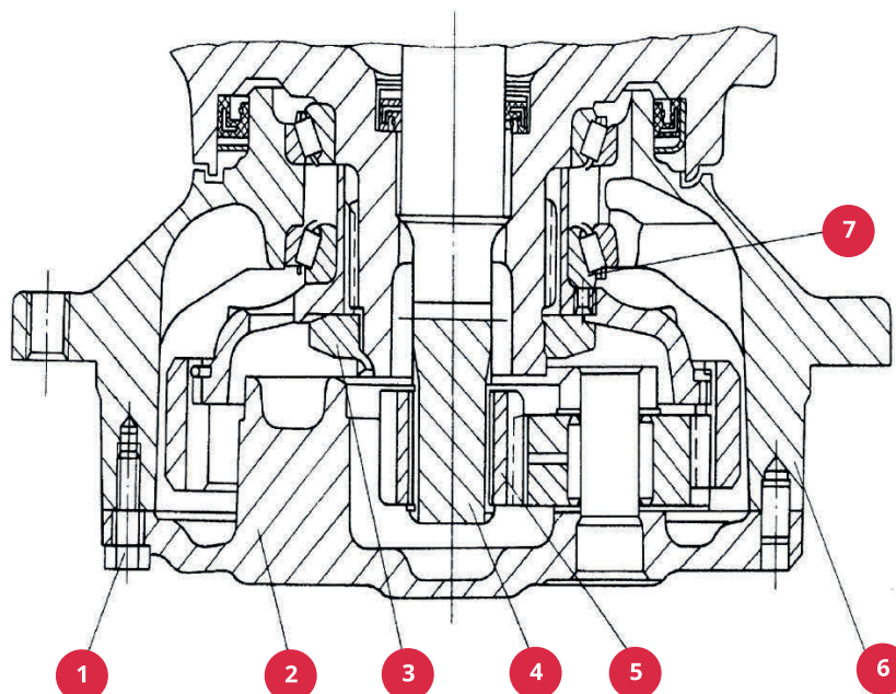
Рис. 2-26. Регулировка колесного редуктора переднего ведущего моста
