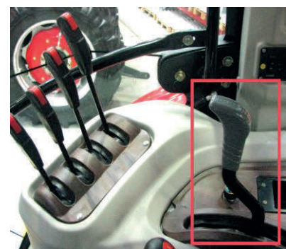
Рис. 2-53. Рычаг управления гидравлической системой
