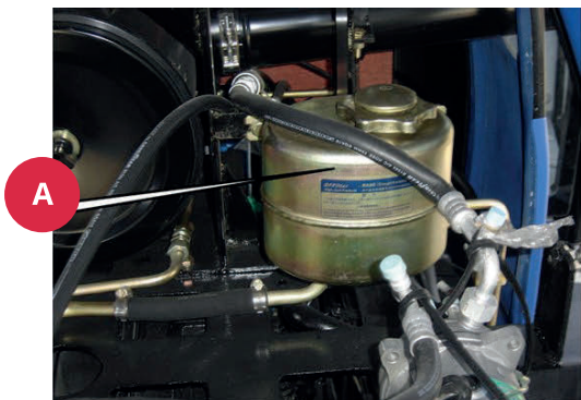
Рис. 2-21. Проверка уровня масла в баке системы рулевого управления
